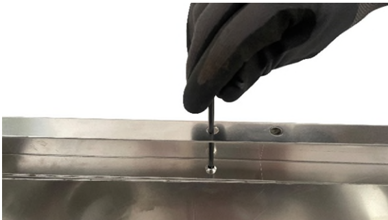
Abbildung 1: Aufstockelemente befestigen
