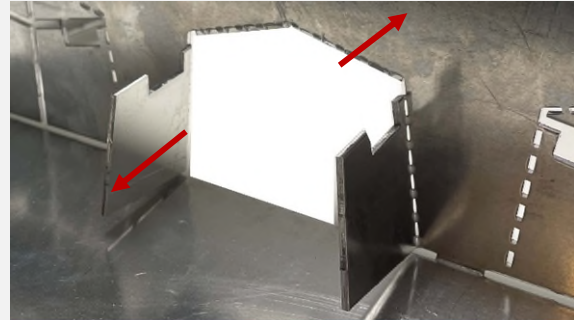
Abbildung 5: Kombianschluss aufbiegen
